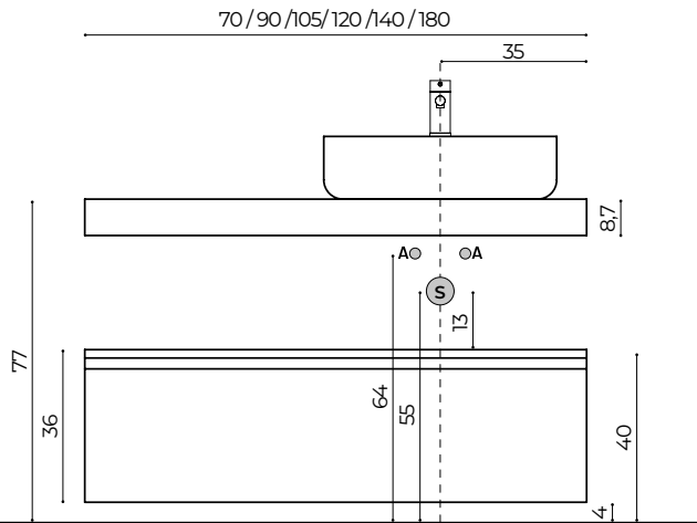
QUOTE PER TOP SCATOLARI CON BASI H.36 QUOTAS DISCHARGES FOR BOX-SHAPED WITH BASE UNIT H. 36
