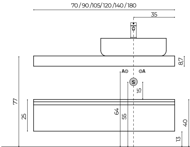
QUOTE PER TOP SCATOLARI CON BASI H.25 QUOTAS DISCHARGES FOR BOX-SHAPED WITH BASE UNIT H. 25
